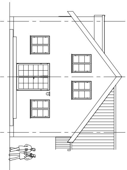
Facade nord
