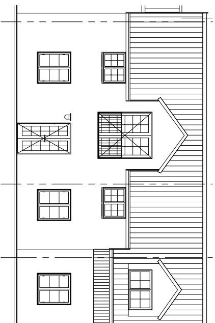
Facade øst
