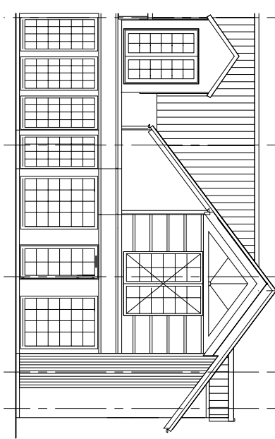
Facade Syd
