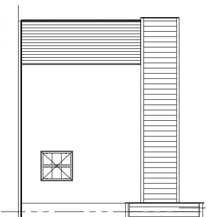
Facade øst
